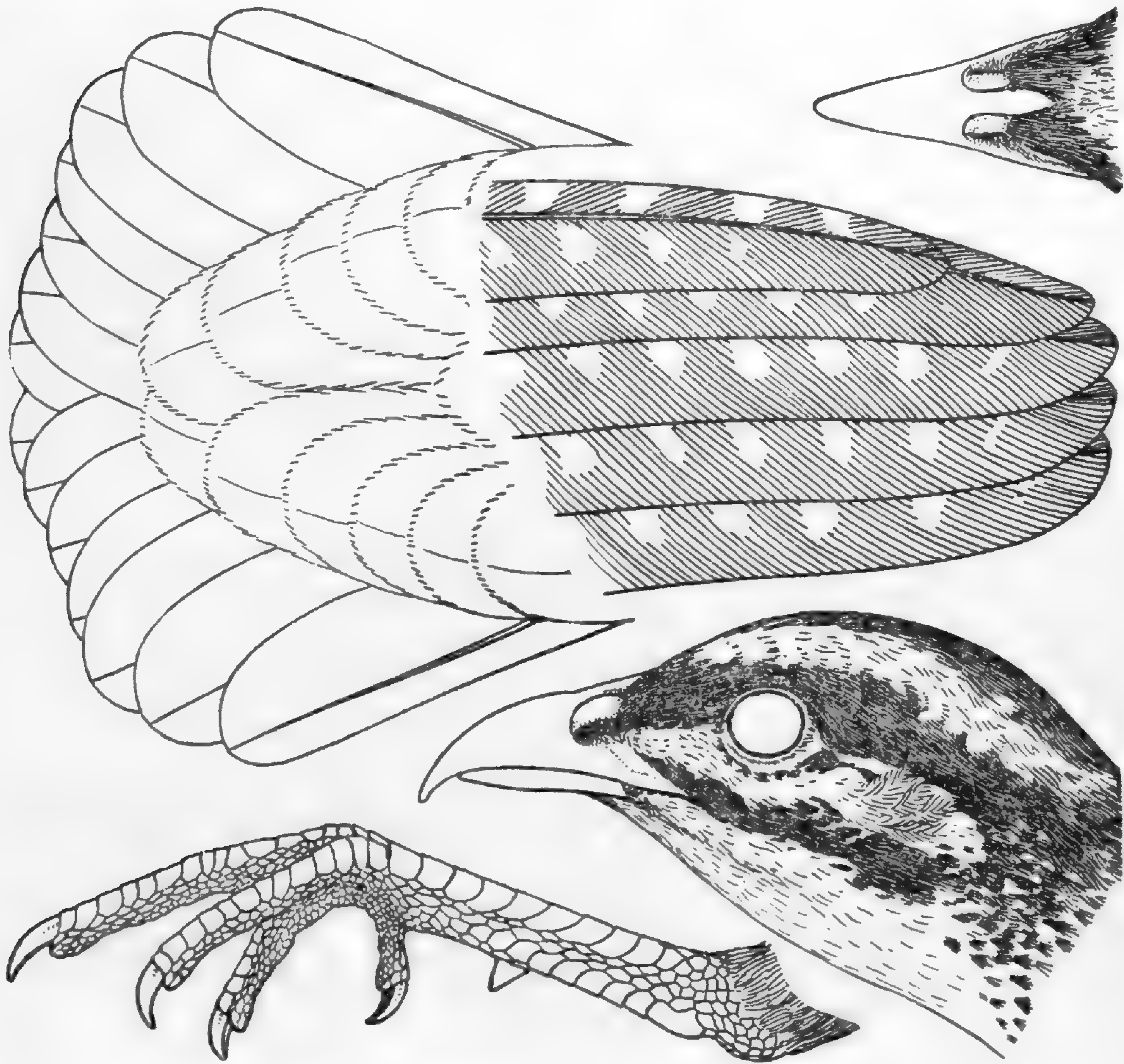
FIG. 1. Francolinus pintadeanus (Scopoli); generic details, \times 1 .
